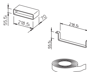
Etrier de fixation Type FB N° Réf. 0626
