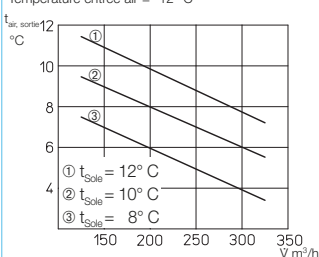
Température sortie air hiver Température entrée air = -12 °C
