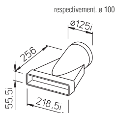
Raccord mixte ø sur Type FUE 100 N° Réf. 0628 Type FUE 125 N° Réf. 0639
