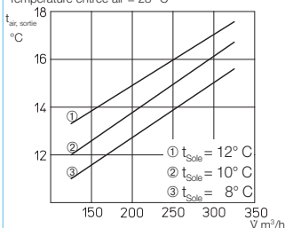
Température sortie air été Température entrée air = 28 °C
