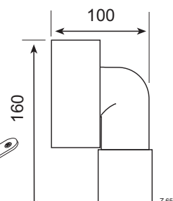
Contre-prise pour prise d'aspiration DISAN
