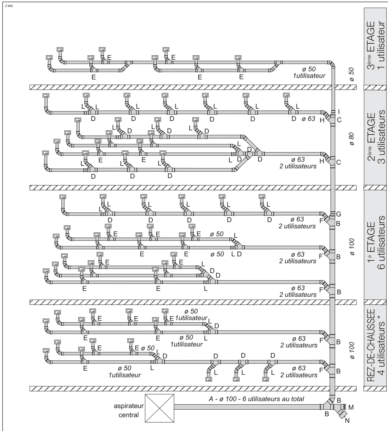
Schéma de répartition du réseau de tuyaux d'aspiration dans une installation comprenant 6 utilisateurs simultanés
