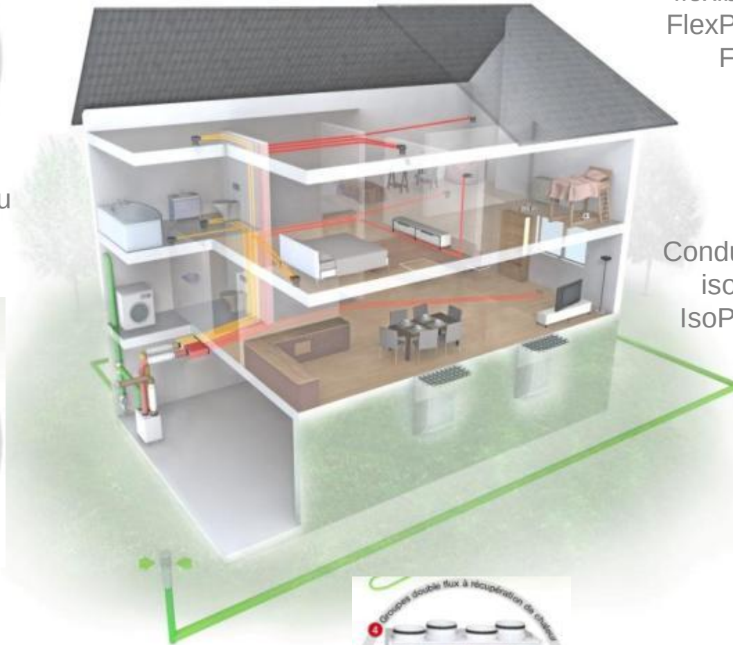
Puits canadien à air LEWT
